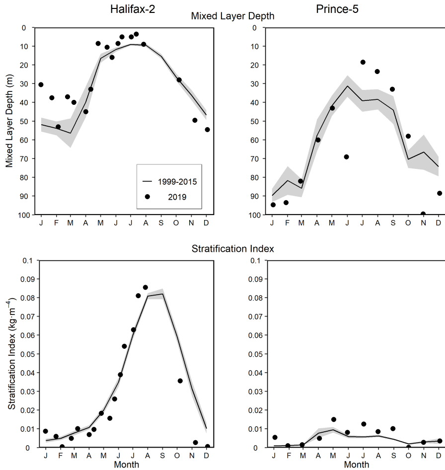
Propriétés de mélange (profondeur de la couche mélangée, indice de stratification) aux stations fixes des Maritimes comparant les données de 2019 (cercle plein) aux conditions moyennes de 1999-2015 (trait plein). La bande ombragée représente l'erreur standard des moyennes mensuelles. Les graduations sur les axes horizontaux indiquent le 15e jour du mois.
